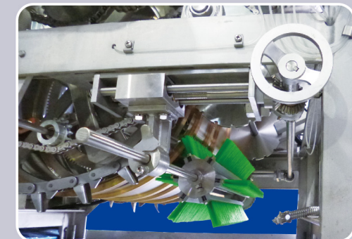
ドラム洗浄ブラシ DRUM CLEANING BRUSH
