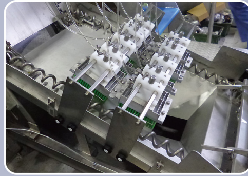
ハンドル式除肉ブラシ SKEWER CLEANING BRUSH
