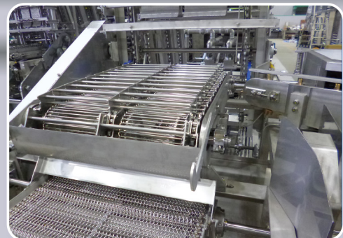
串抜き SKEWER PULLER
