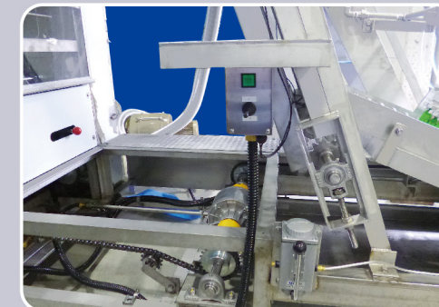
電磁クラッチ ELECTROMAGNETIC CLUTCH
