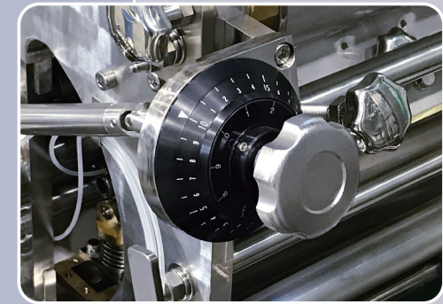
ダイヤル式目付調整 WEIGHT ADJUSTMENT DIAL
