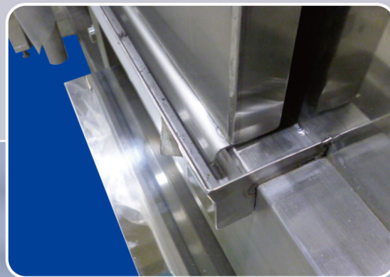
ウォーターシール WATER SEAL サイドからの 蒸気もれがない。
