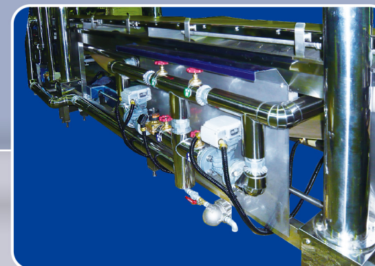
温度比例制御(低圧の省エネタイプ) PLC TEMPERATURE CONTROLLER
