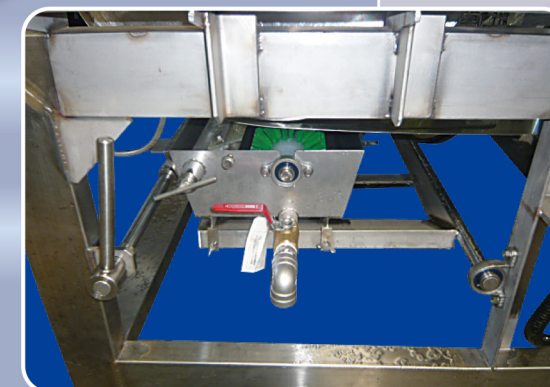
洗浄装置(テフロンベルト式) CONVEYOR WASHER
