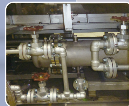
熱交換機(循環式フライヤーのみ) HEAT EXCHANGER
