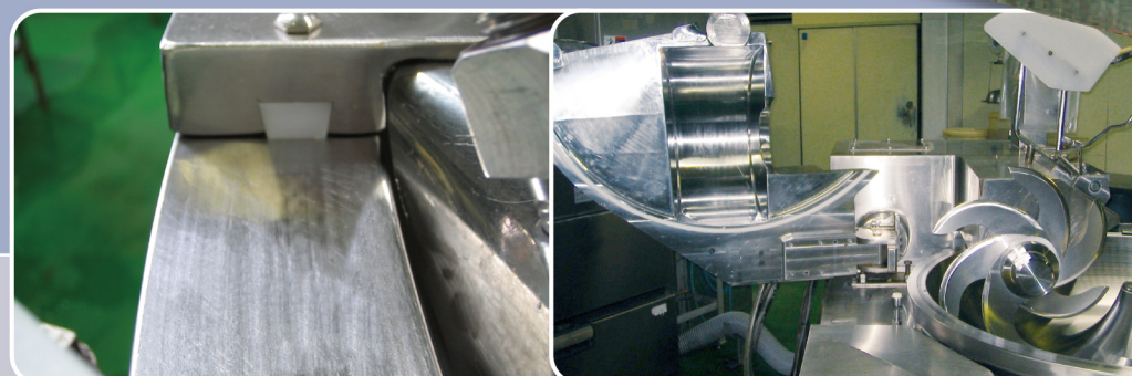
肉もれ防止板 BLADE COVER GUIDE 床への飛び散り防止で衛生的。
