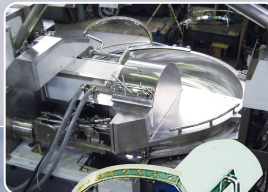
刃物洗浄装置 CIP ASSIST 刃物自動洗浄で安全
